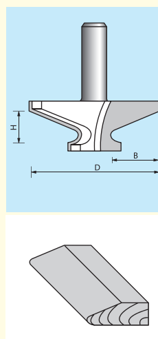
2015 TABLE EDGE BIT 水鴨咀刀
