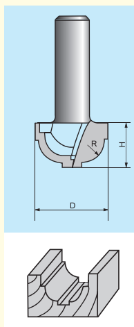
0704M FLAT OGEE BIT WITHOUT BEARING 雙邊平台曲線刀 (沒有軸承作導向)
