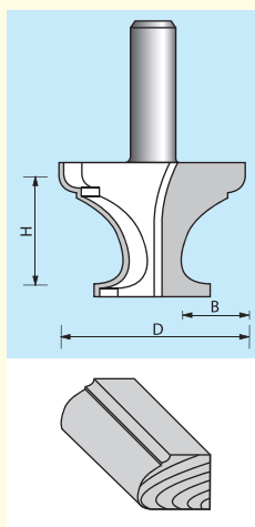
2013 TABLE EDGE BIT 仍鈎刀
